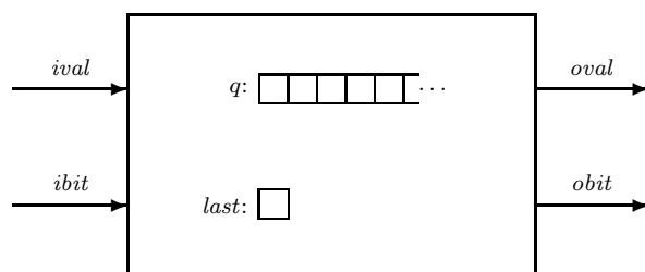
Fig. 1. A simple queue.
